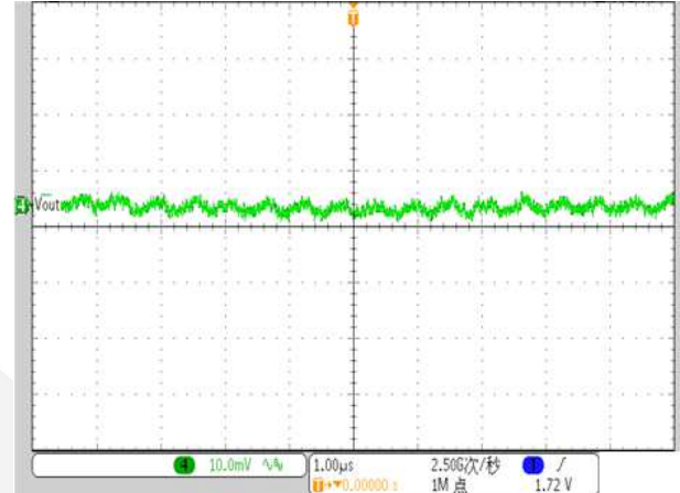
Ripple (Iload=1.2A)
