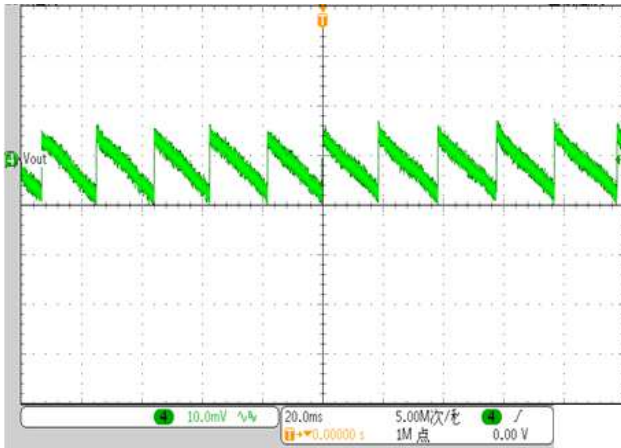
Ripple (Iload=0A)
